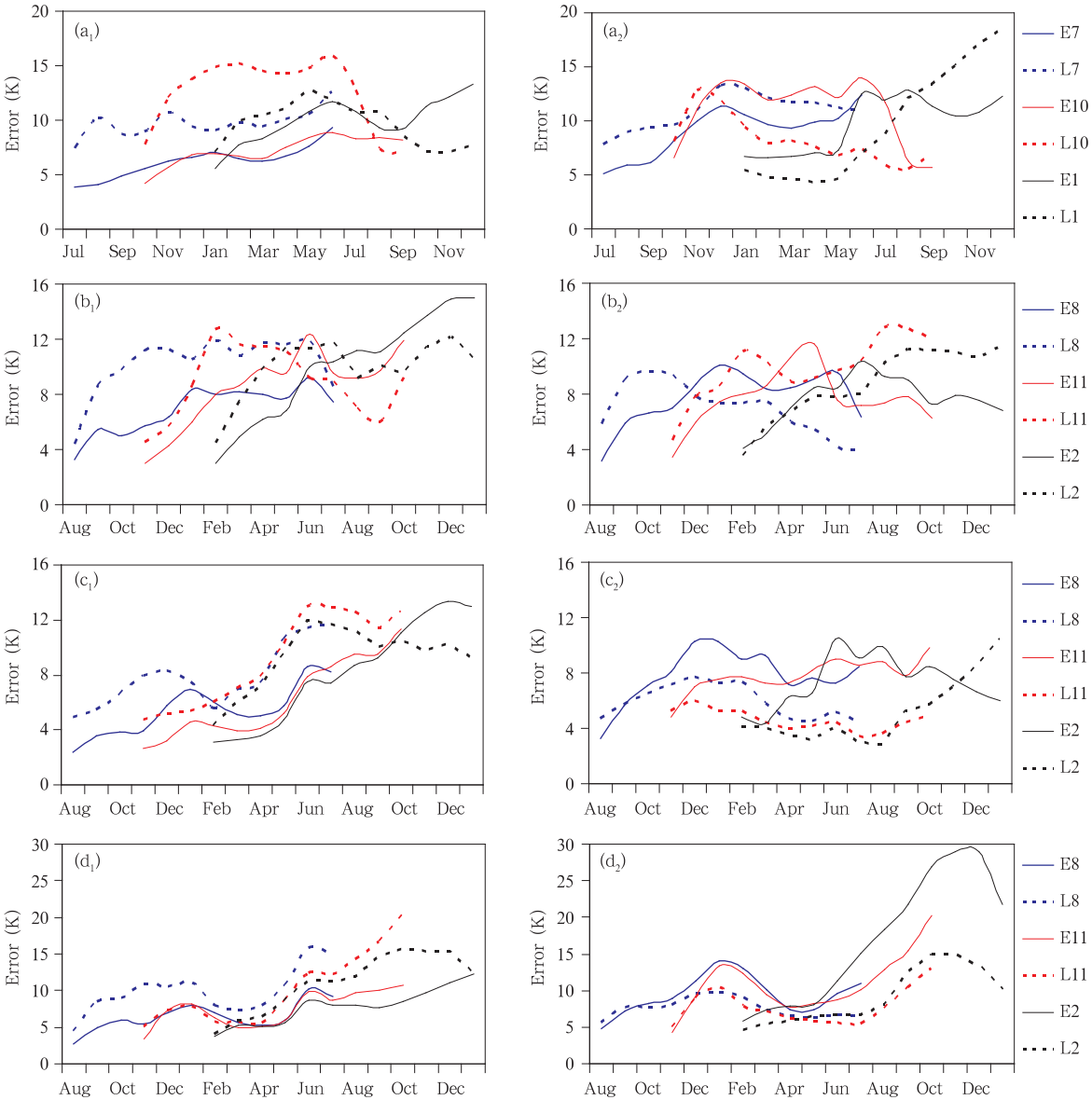
图 5 模式预报 ENSO 事件生长期( a_1-d_1 )和衰减期( a_2-d_2 )的逐月预报误差 (a. FGOALS 模式, b. GFDL 模式, c. SNU 模式, d. UH 模式;实线为厄尔尼诺事件,E8 指厄尔尼诺事件,8 月起报,其他同; 虚线为拉尼娜事件,L8 指拉尼娜事件,8 月起报,不同颜色代表不同起报月)
