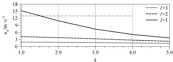
图 11 给定不同经向波数下由公式 (6) 计算得到的特征风速 (m/s) 随 k 的变化曲线
