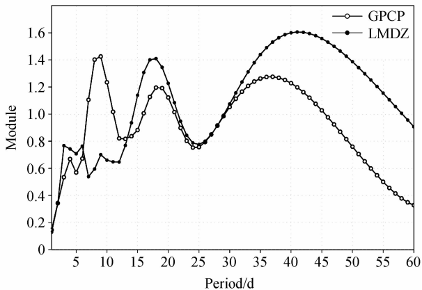
图 5 同图 1, 但为降水
