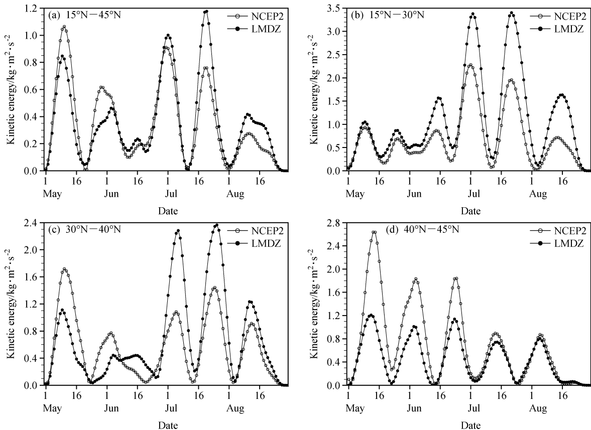
图 4 30~60 天带通滤波后沿 105°E~122.5°E 平均的 850 hPa 动能随时间变化 (单位: \text{kg} \cdot \text{m}^2 \cdot \text{s}^{-2} ): (a) 15°N~45°N; (b) 15°N~30°N; (c) 30°N~40°N; (d) 40°N~45°N
