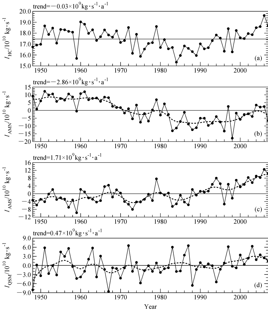
图 2 (a) Hadley 环流强度指数 I_{HC} 、(b) 北半球非对称模态指数 I_{AMN} 、(c) 南半球非对称模态指数 I_{AMS} 以及 (d) 对称模态指数 I_{QSM} 的时间序列 (单位: 10^{10} kg/s)。虚线: 各时间序列 9 年 Gaussian 滤波的结果 Fig. 2 The time series of (a) I_{HC} , (b) I_{AMN} , (c) I_{AMS} , and (d) I_{QSM} (units: 10^{10} kg/s). The 9-year Gaussian filtered results (dashed lines) are also shown in (b)–(d)
