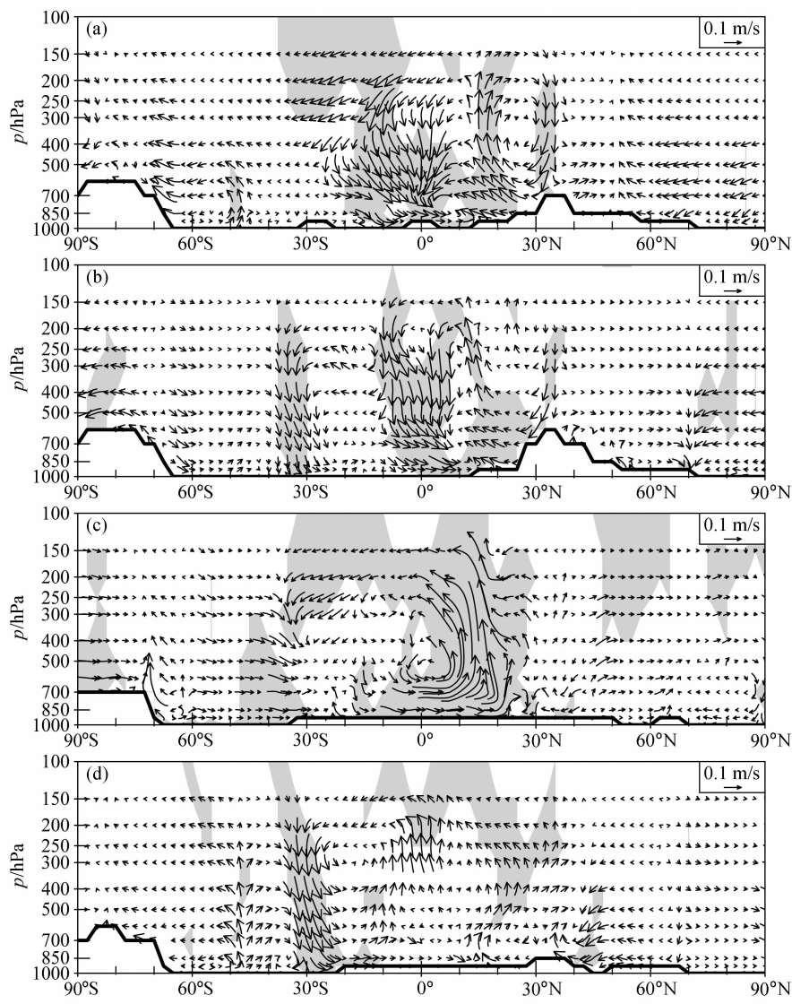
图 7 (a) SCSSM、(b) SASM2、(c) WASM、(d) SASM1 对应经度范围内纬向平均垂直环流在高低季风指数年份的合成差分析。阴影表示合成的风场至少有一个分量超过 95% 信度检验
